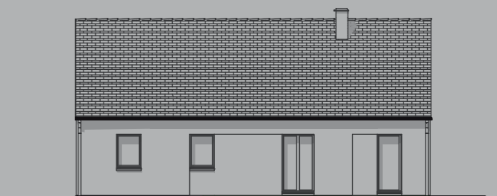
FAÇADE SUD - éch: 1/200
